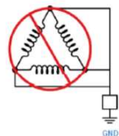
Transformateur de mise à la terre
